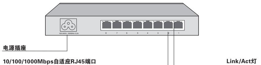
图1-2 TL-SG1008后面板示意图
